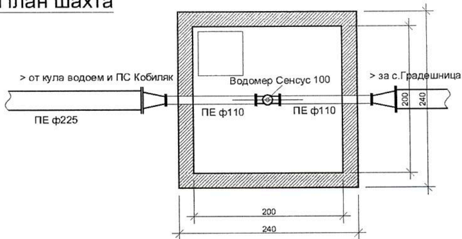
План шахта
